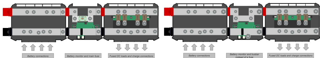
Zusammengeschnittene Lynx-Module: Lynx Power In, Lynx Shunt VE.Can und Lynx Distributor. Rechts die Variante M10 mit Sammelschiene anstelle der Sicherung
